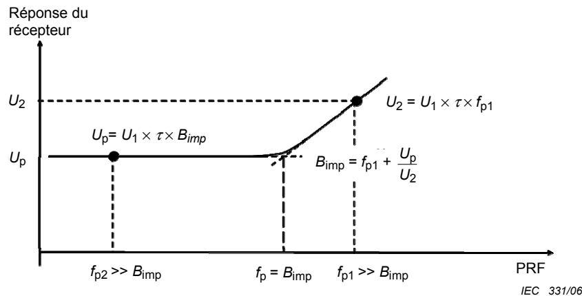
Figure E.7 – Calcul de la largeur de bande d'impulsion
