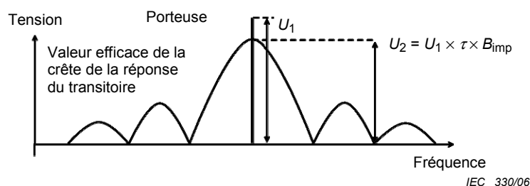
Figure E.6 – Filtrage avec une B_{imp} nettement plus large que la prf
